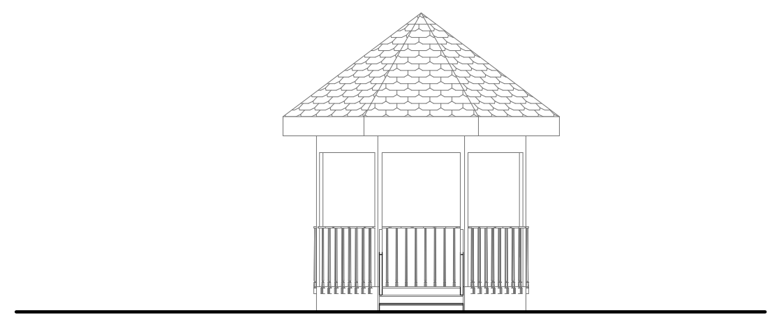
D.2 RAMADA NORTH ELEVATION SCALE: 1/8" = 1'-0"
