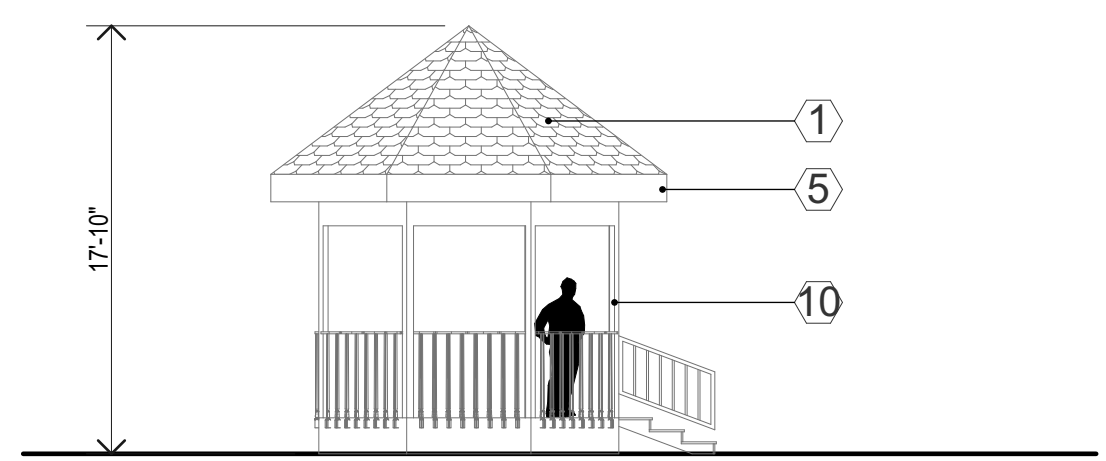
D.1 RAMADA EAST ELEVATION SCALE: 1/8" = 1'-0"
